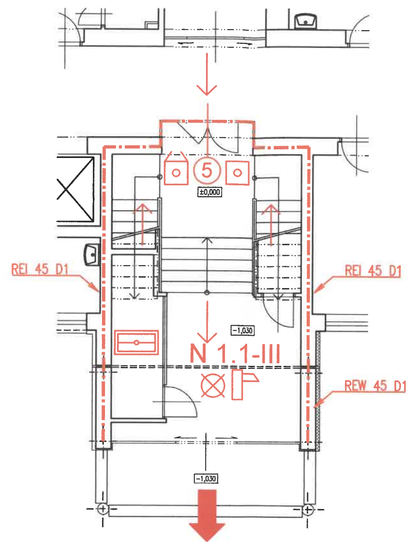
PŮDORYS I.NP - NOVÝ STAV
