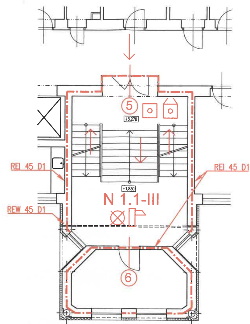
PŮDORYS II., III, IV.NP - NOVÝ STAV
